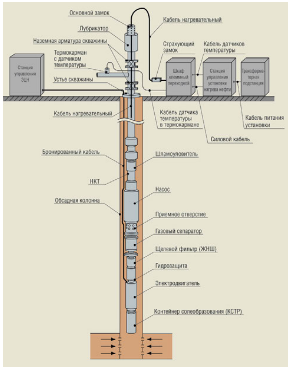
Принципиальная компоновка оборудования электроцентробежного насоса для нефтяных скважин Уренгойского месторождения
