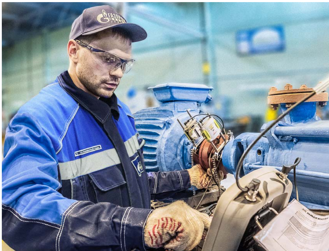
Игорь Мошкин, слесарь-ремонтник Управления аварийно-восстановительных работ, выполняет центровку валов электронасосного агрегата
